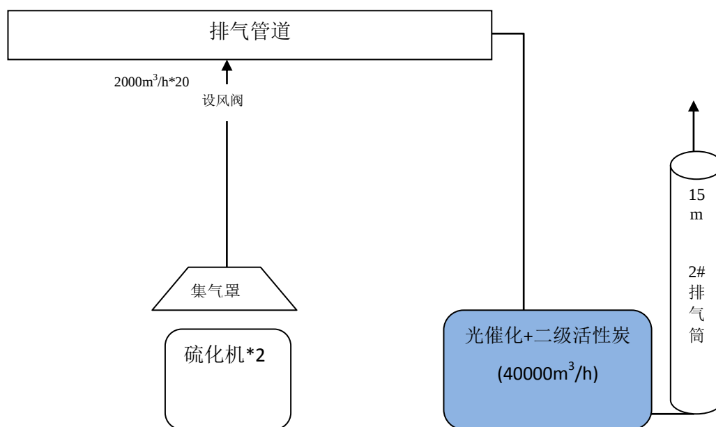
图 2.2-8 硫化废气收集与处理措施图
