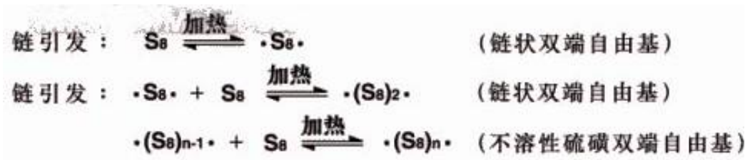
图 2.2-4 硫磺反应机理图
