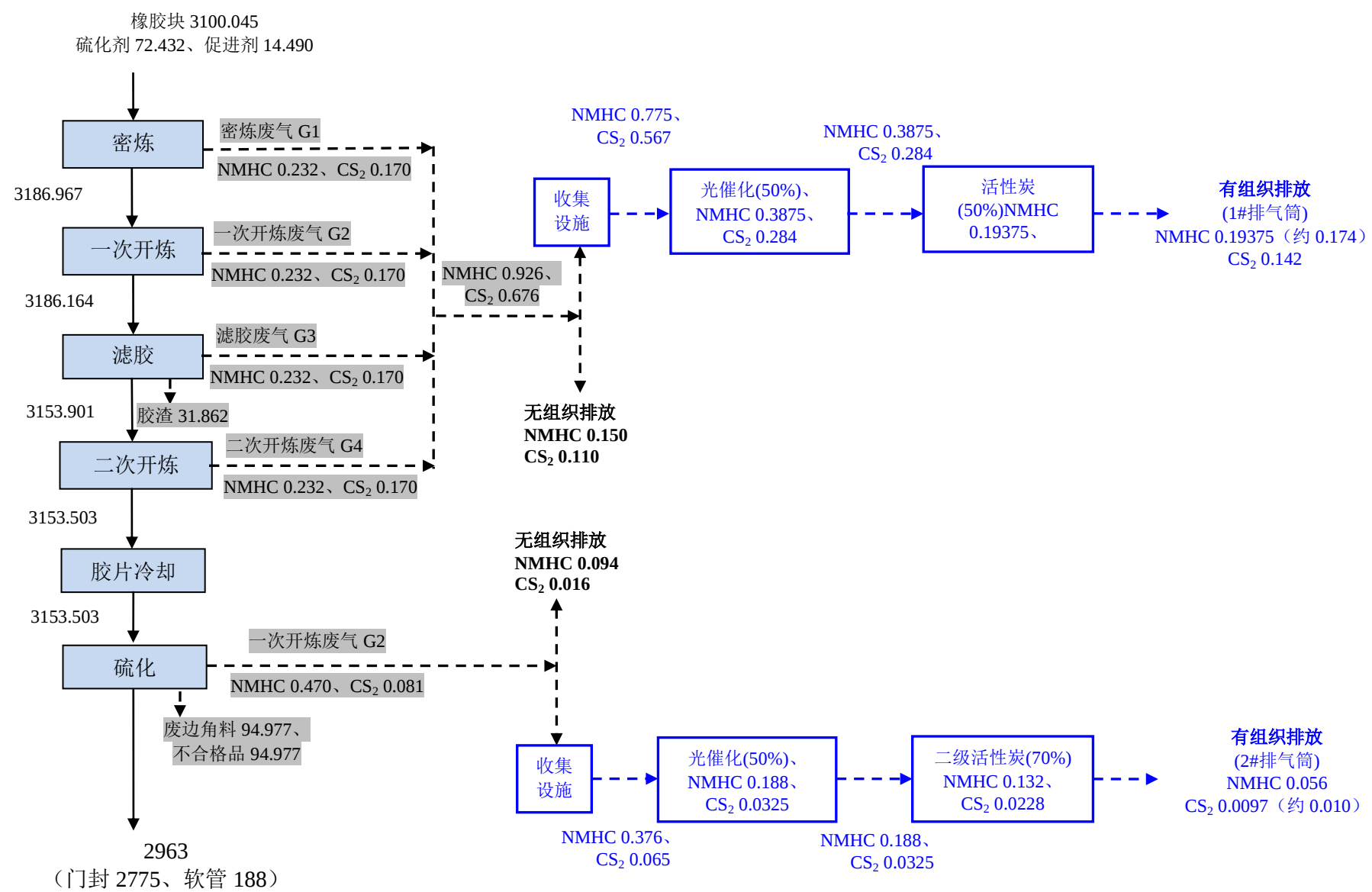
图 2.2-6 橡胶产品物料平衡图 (t/a)
