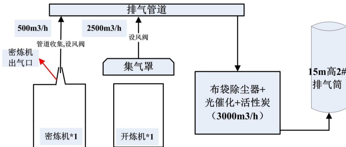
图 6.1-2 密炼废气、滤胶废气、开炼废气处理示意图
