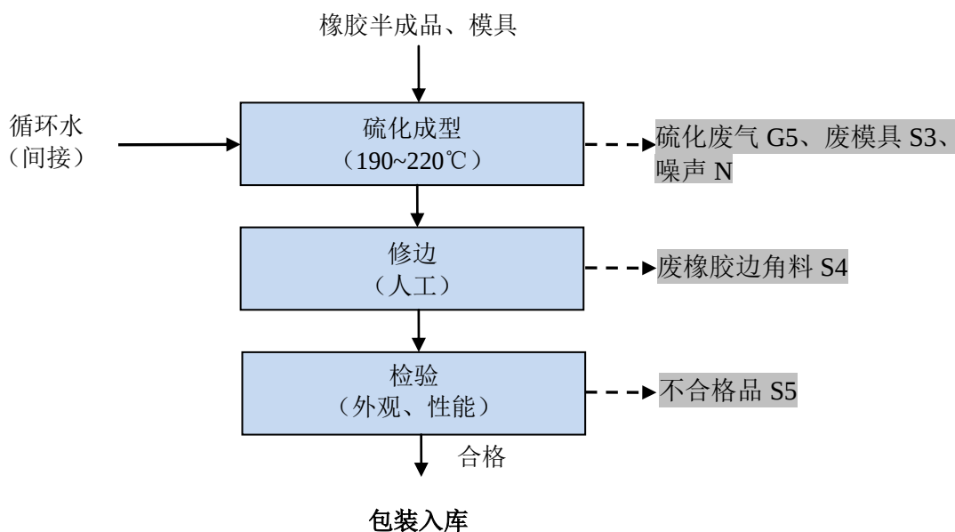
图 2.2-3 纯橡胶产品生产工艺流程及产污环节图
