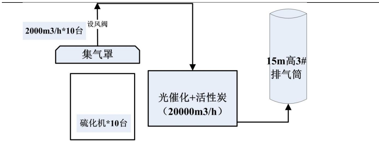
图 6.1-3 硫化废气处理示意图（最大开启 20 台硫化机）
