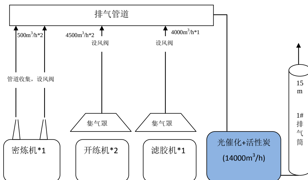
图 2.2-7 密炼废气、开炼废气、滤胶废废气收集与处理措施图
