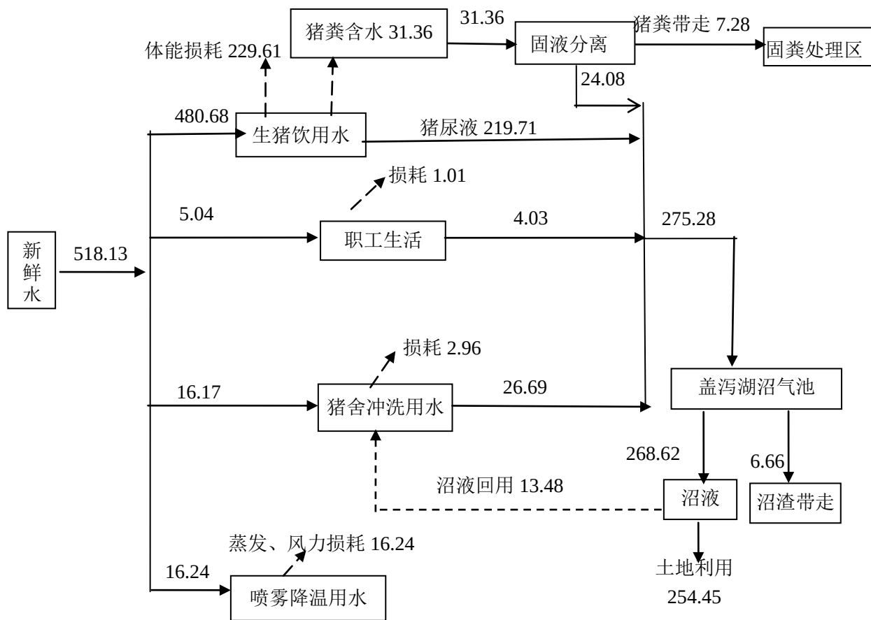
图 2-11 项目夏季水平衡图 (122 天, 单位: \text{m}^3/\text{d} )
