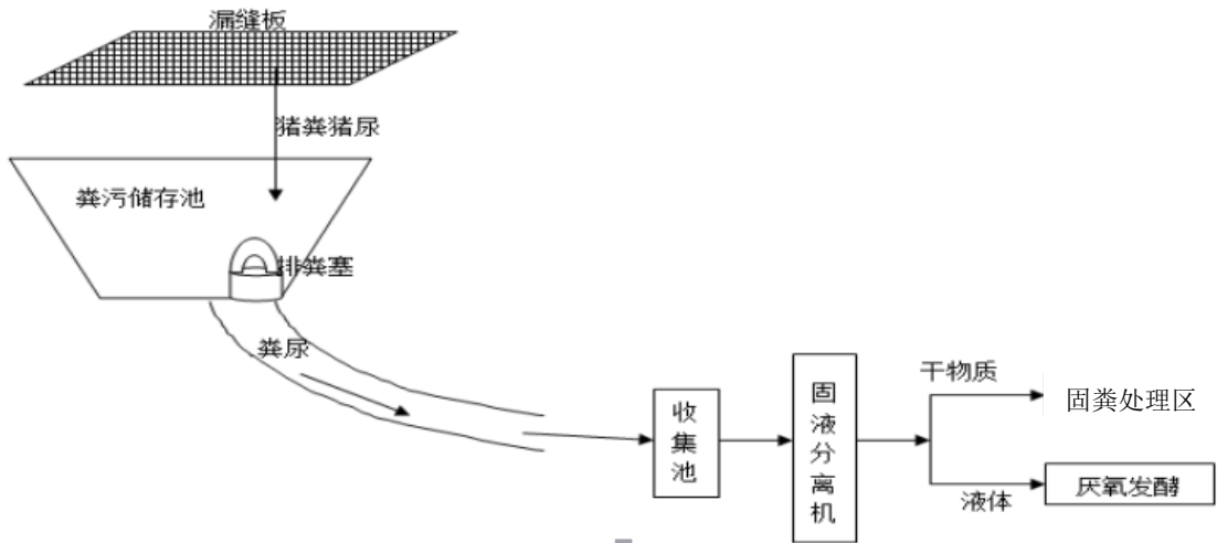
图 2-3 本项目清粪工艺示意图
