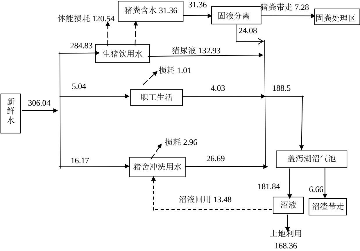
图 2-10 项目春、秋、冬季水平衡图（243 天，单位：m³/d）
