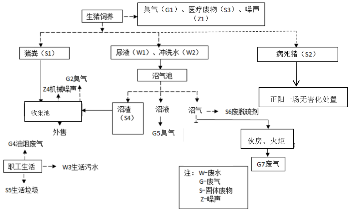
图 2-9 产污环节图
