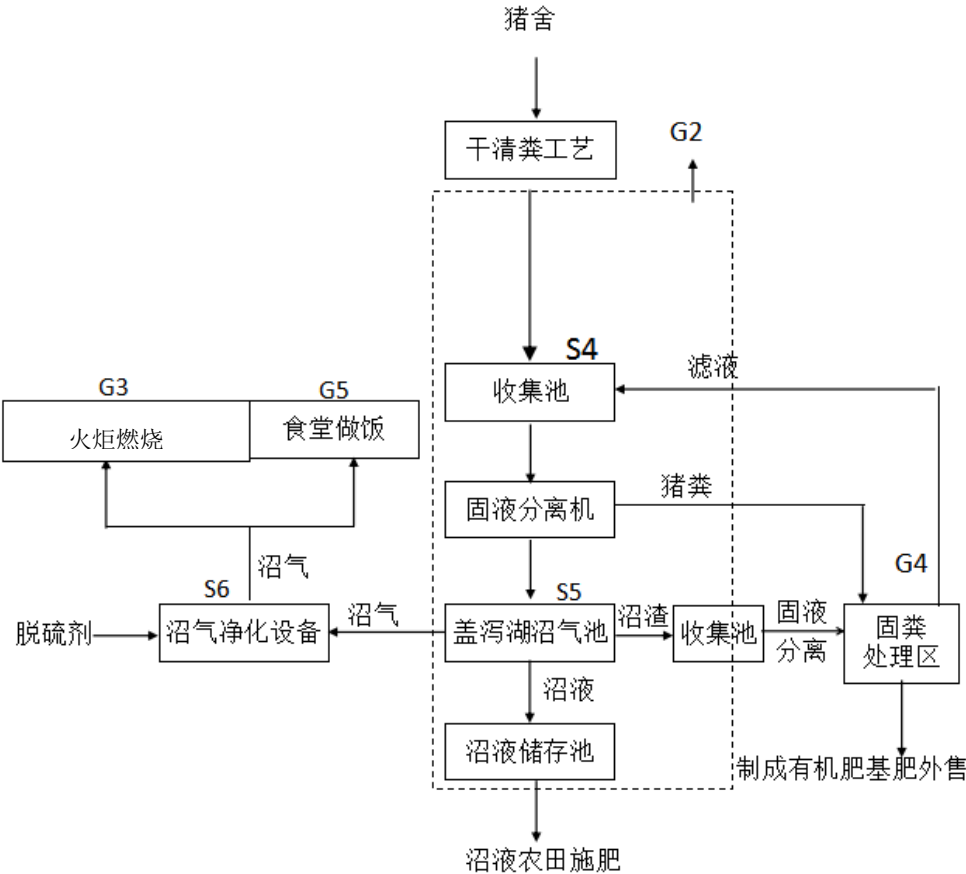
图 2-4 项目污水处理工艺流程图
