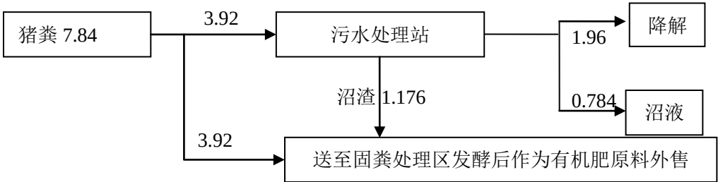
图 2-13 项目猪粪、沼渣平衡图单位：干 t/d
