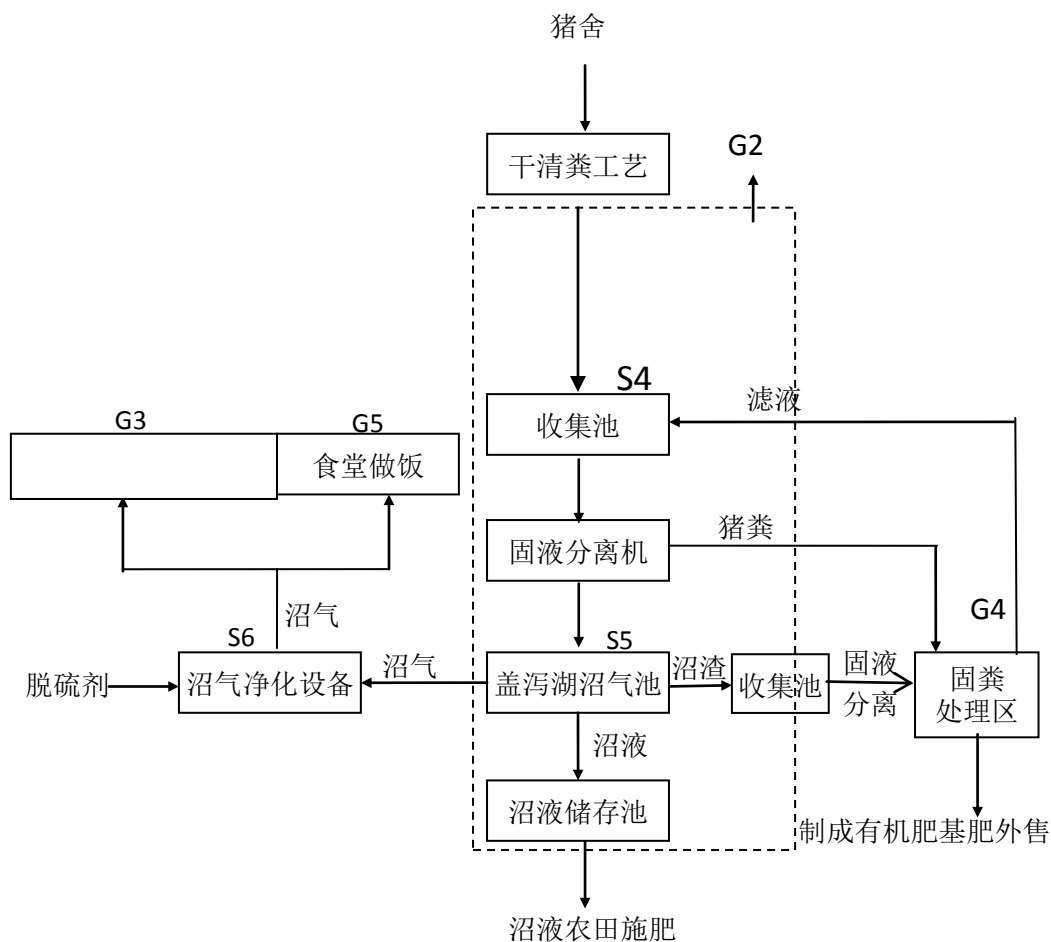
图 5-1 工程污水处理工艺流程图
