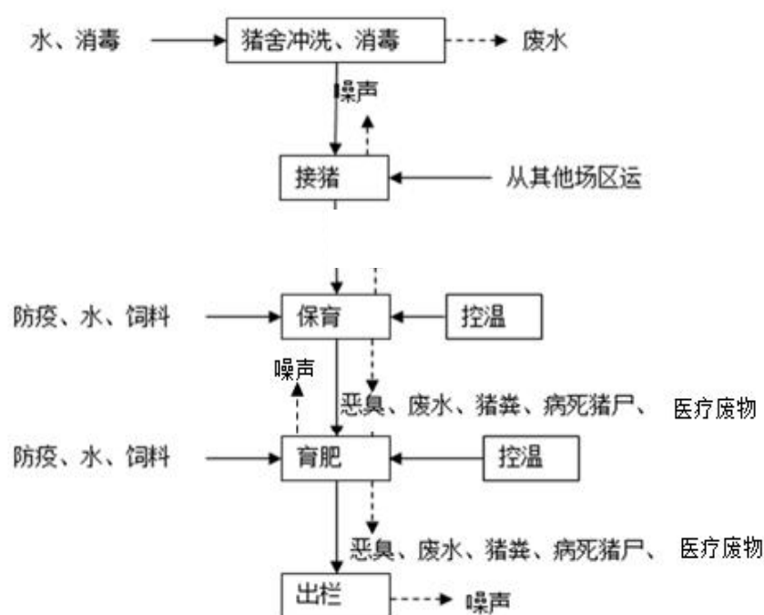
图 2-2 后备养殖过程工艺流程及产污环节图
