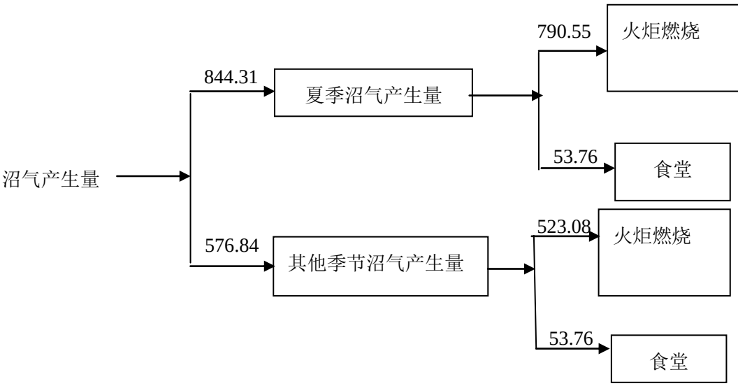
图 2-6 沼气利用平衡图 单位：m³/d
