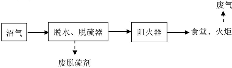
图 2-5 沼气利用流程及产污环节图
