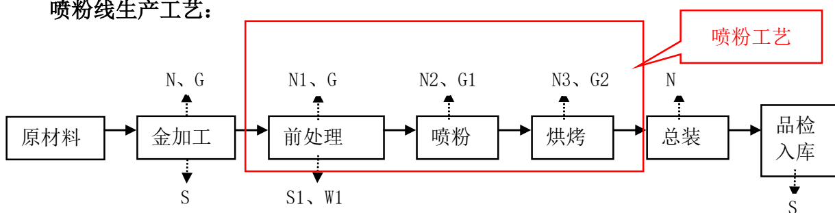
图4.2-3 喷粉线生产工艺流程图
