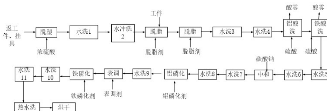
图4.2-5 外前处理生产工艺流程图
