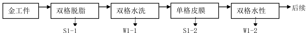
图4.2-4 项目内前处理工艺流程图
