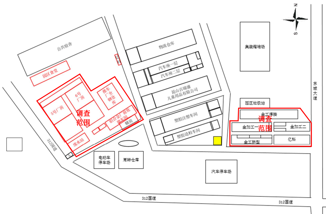
图 4.1-1 好孩子儿童用品有限公司5~11号厂房平面布置图
