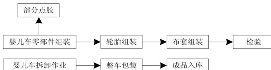
图4.2-1 婴儿推车生产工艺流程图
