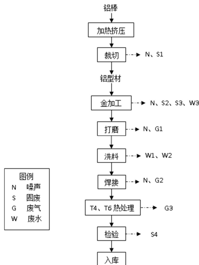
图4.2-2 铝合金厂生产工艺流程图
