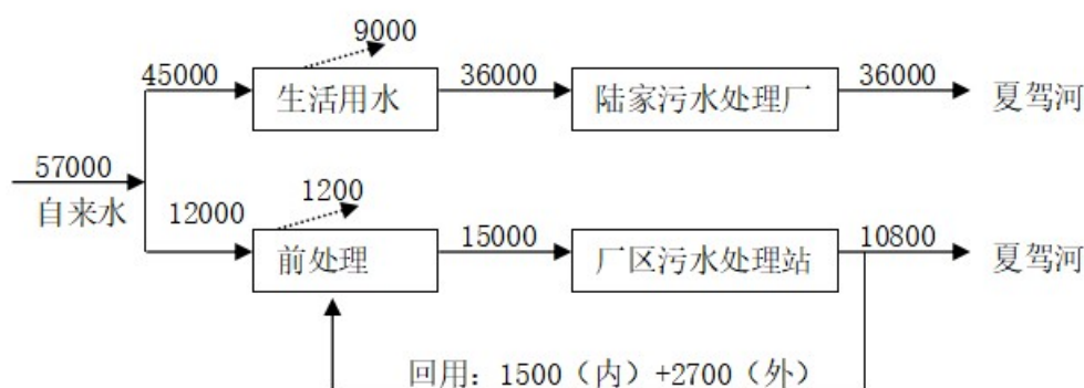
图 4.2-5 推车厂全厂水量平衡
