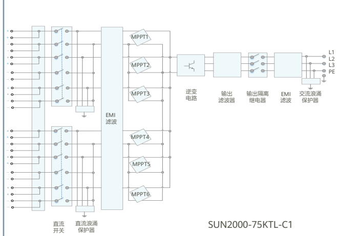
电路框图
