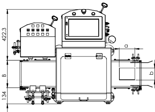
顶视图
