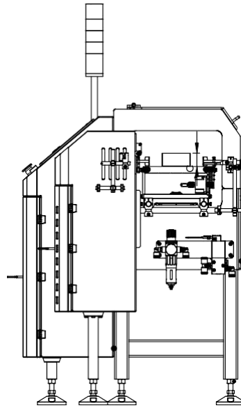
侧视图
