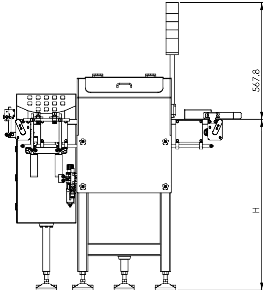
正视图
