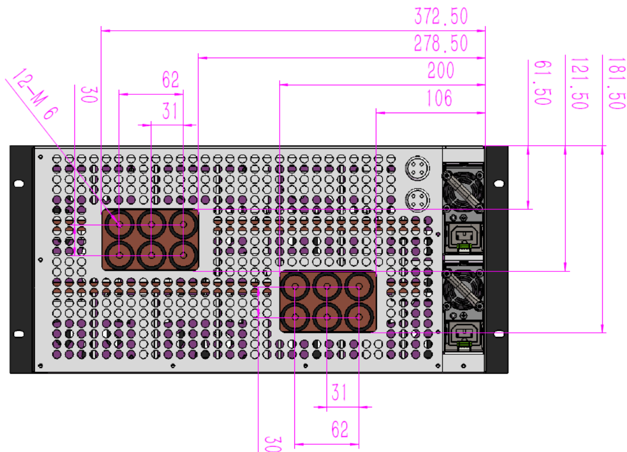
图 5 后面板
