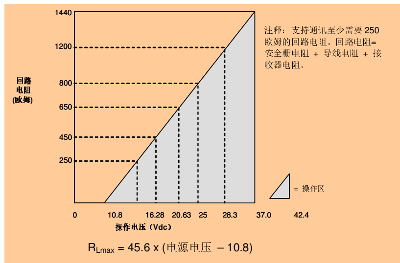
图 2 - 电源电压和回路电阻图及计算
