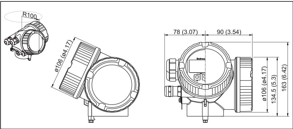
GT19 外壳 (塑料 PBT) ; 单位: mm (in)
