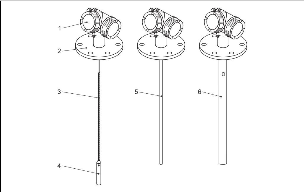
Levellflex 的结构设计图
