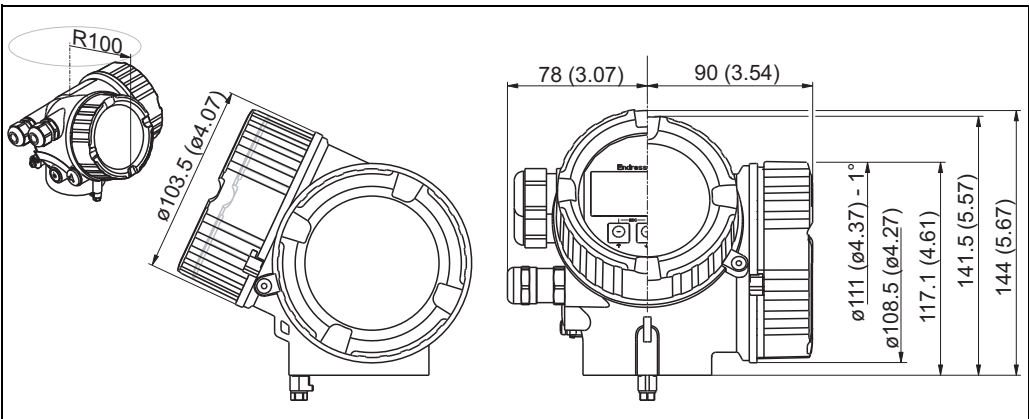
GT20 外壳 (铝, 带涂层) ; 单位: mm (in)
