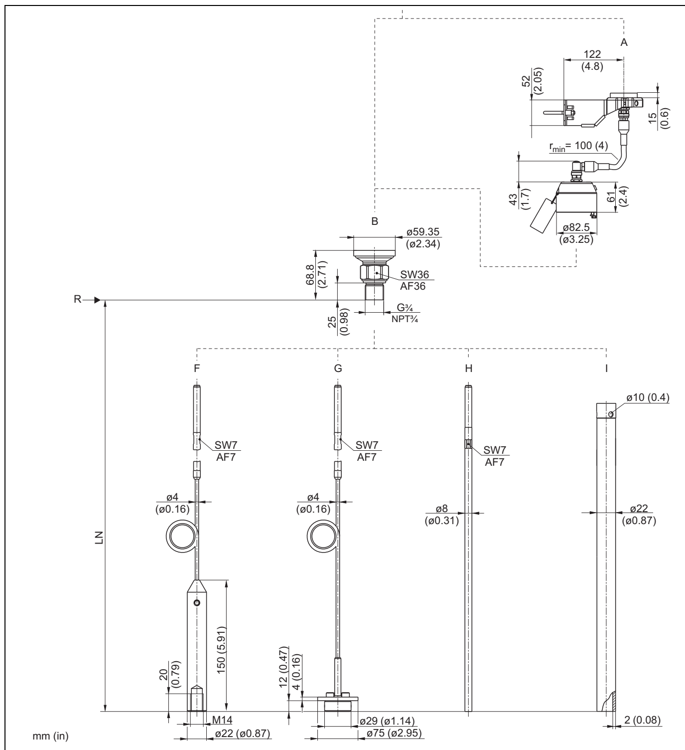
FMP51: 过程连接 (G \frac{3}{4} 、NPT \frac{3}{4} ) 和探头的外形尺寸
