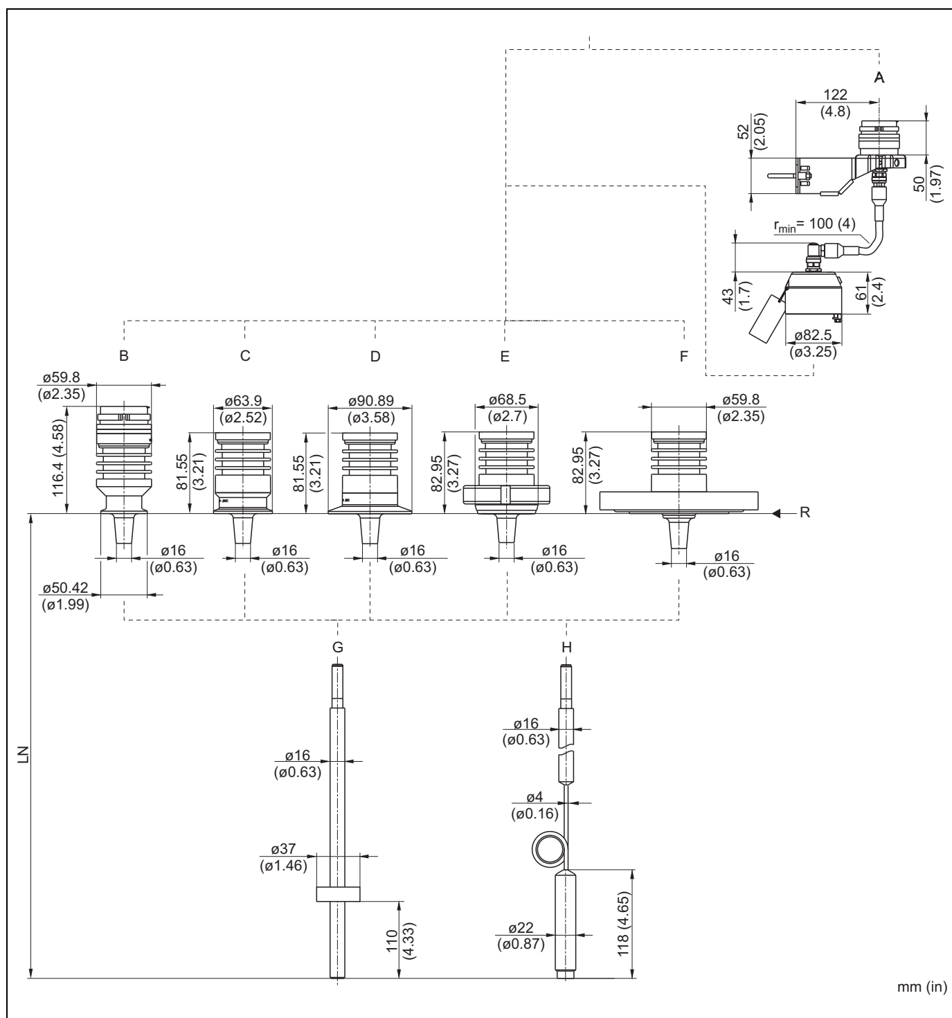
FMP52: 过程连接和探头的外形尺寸
