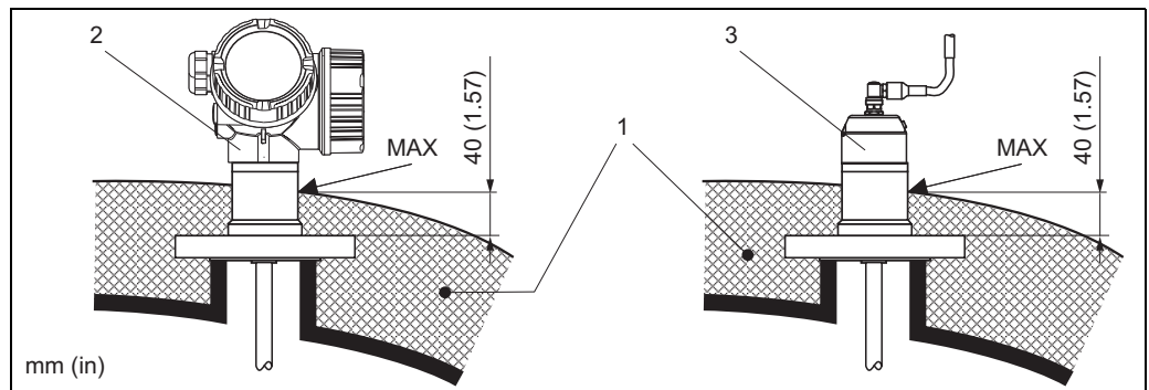
带法兰过程连接的 FMP51 和 FMP52
