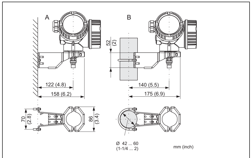
电子接线腔外壳的安装支架的外形尺寸示意图
