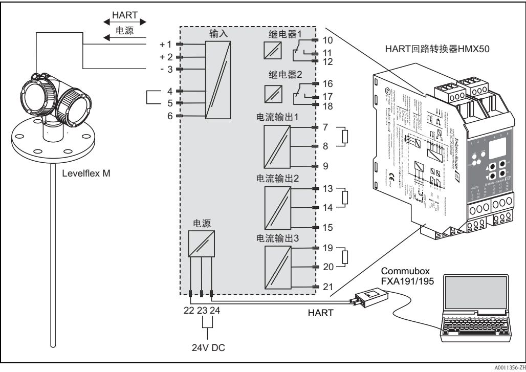
与 HART 回路转换器 HMX50 的连接示意图 (例如：两线制无源设备和电流输出的连接示意图)
