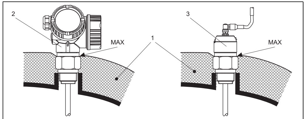
带螺纹过程连接的 FMP51
