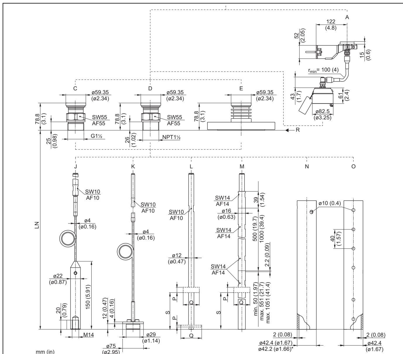
FMP51: 过程连接 (G1½、NPT1½、法兰) 和探头的外形尺寸
