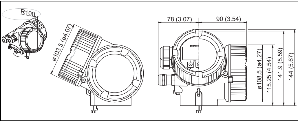
GT18 外壳 (316L) ; 单位: mm (in)
