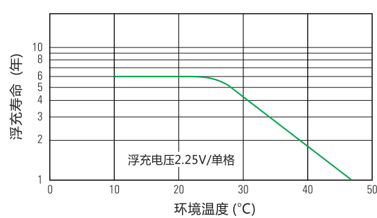
浮充寿命曲线
