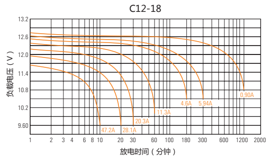
放电特性曲线
