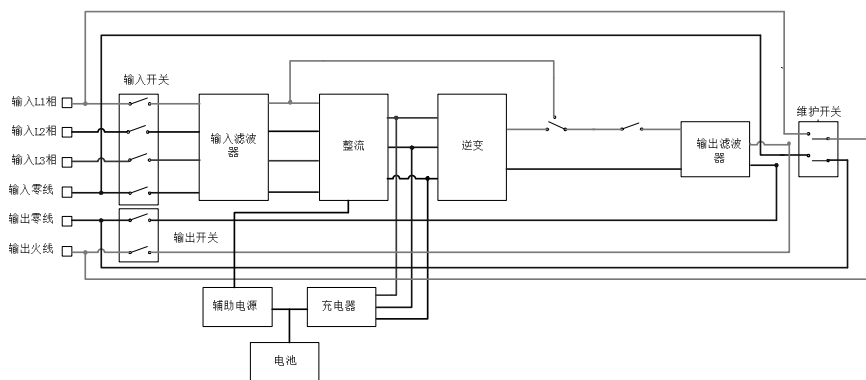
9E15KCXL/9E20KCXL 电气框图
