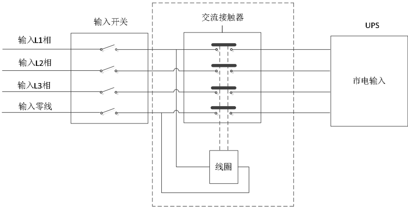
典型外部隔离装置安装
