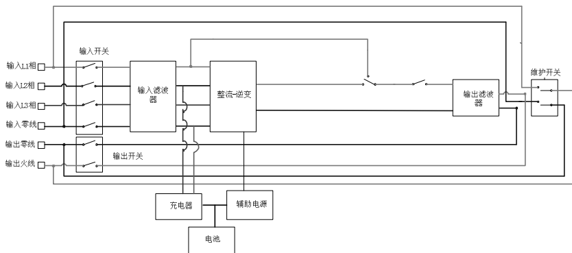
9E10KCN/9E10KCNXL 电气框图
