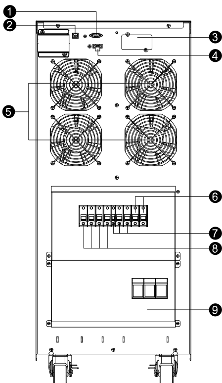
9E15KCNXL/9E20KCNXL 带后面板盖
