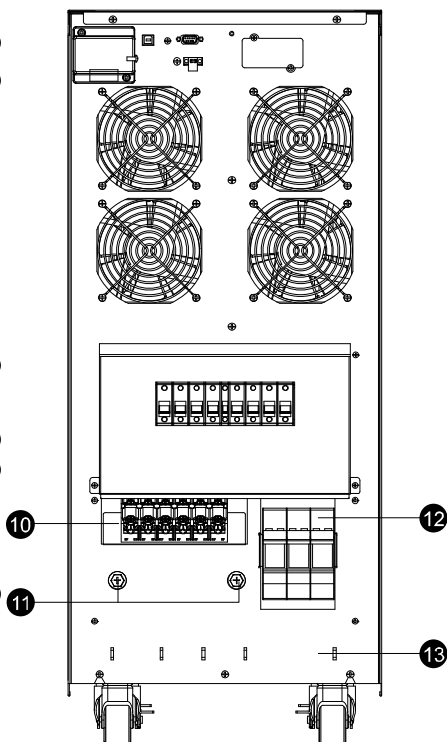
9E15KCNXL/9E20KCNXL 不带后面板盖
