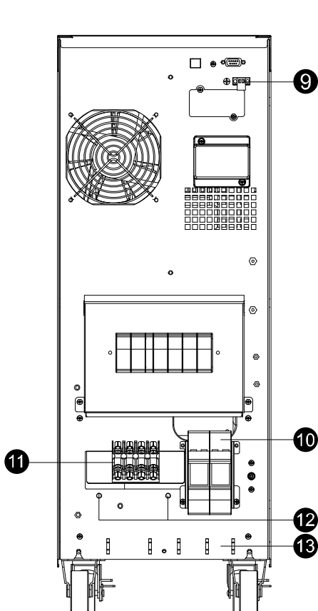
9E6KCN/9E6KCNXL 不带后面板盖
