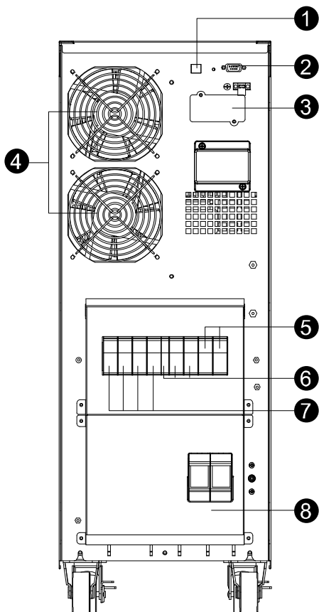
9E10KCN/9E10KCNXL 带后面板盖
