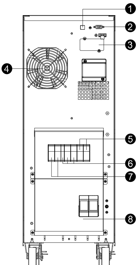
9E6KCN/9E6KCNXL 带后面板盖
