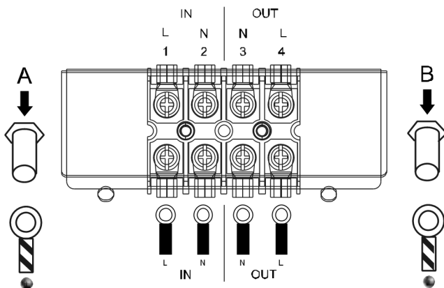
6K端子视图
