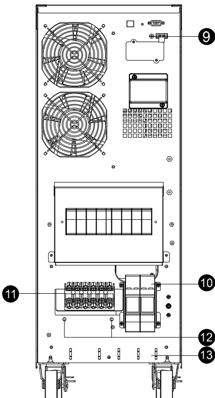
9E10KCN/9E10KCNXL 不带后面板盖
