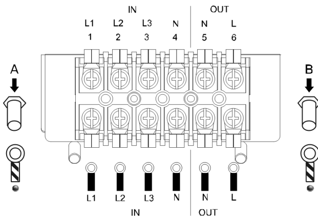
3-6. 10~20K 三相输入端子视图
