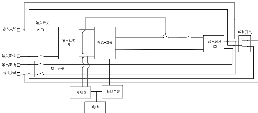
9E6KCN/9E6KCNXL 电气框图
