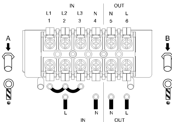
3-5. 10~20K 单相输入端子视图
