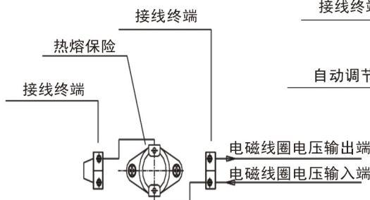
E 1 内部温控 (GTRM-1)
