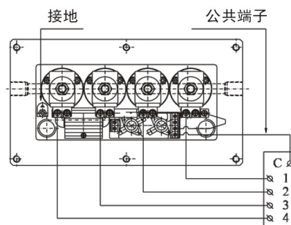
E 2 内部温控和温度调节器 GTRM 2
