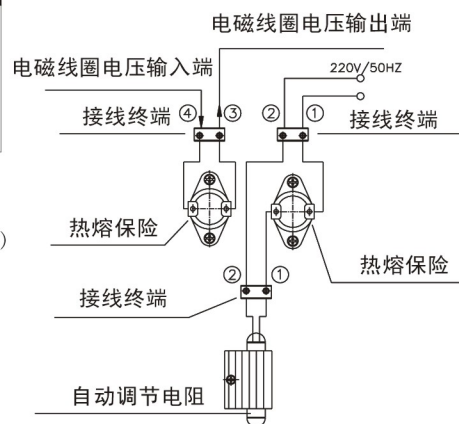
E 2 内部温控和温度调节器 GTRM 2
