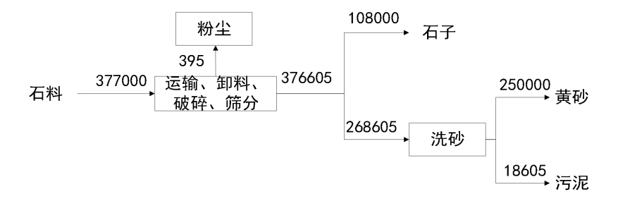
图 2-2 本技改项目物料平衡图 单位 t/a
