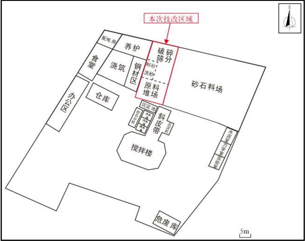
图 2-3 项目厂区平面布置图
