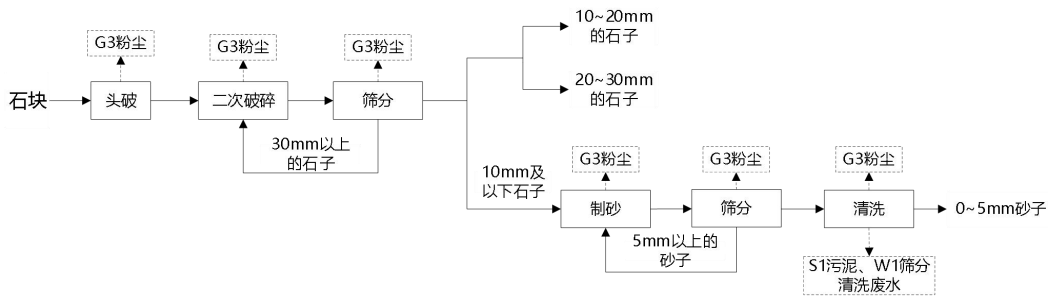
图 2-5 项目生产工艺流程及产污图
