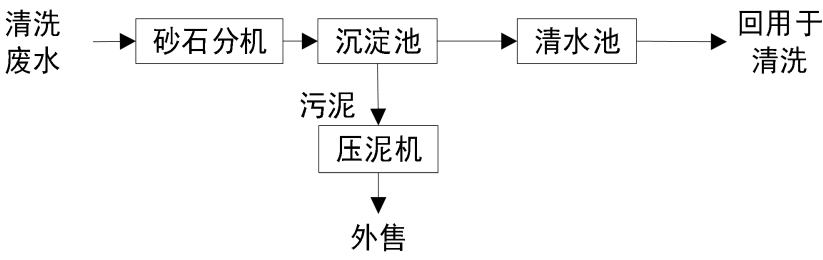
图 4-1 废水处理工艺
