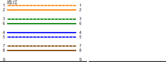
接线图 (T568B)
