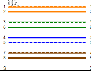
接线图 (T568B)
