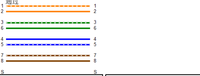
接线图 (T568B)
