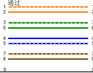
接线图 (T568B)
