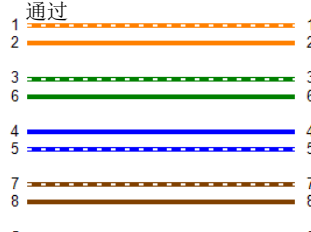
接线图 (T568B)
