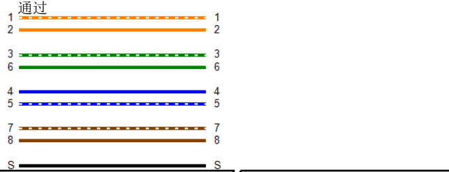
接线图 (T568B)
