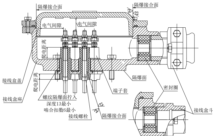
图 2 接线盒结构
