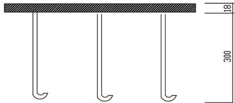
剖面
