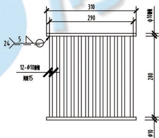
柱详图 2:1
