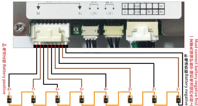
8S接线图 (8S wiring diagram)
