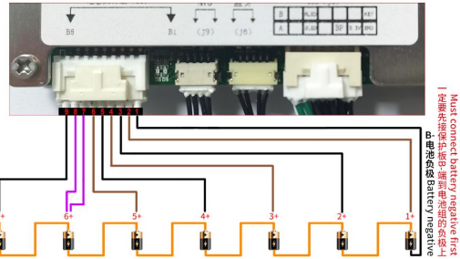
8S接线图 (8S wiring diagram)
