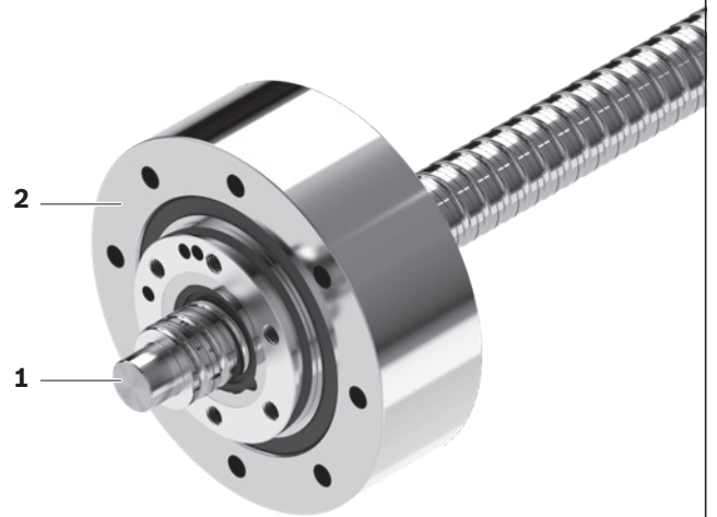
1 滾珠絲杠傳動系統 (BASA)-絲杠 2 被驅動的螺母 FAR
