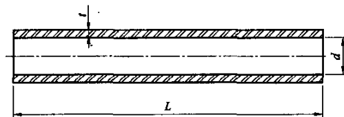
d —公称内径； t —公称壁厚； L —总长
