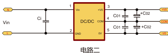
电路二
