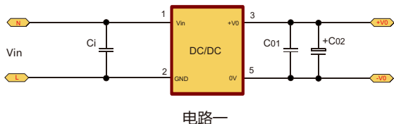
电路一
