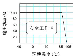
温度曲线图
