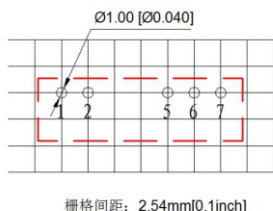
推荐 PCB 图
