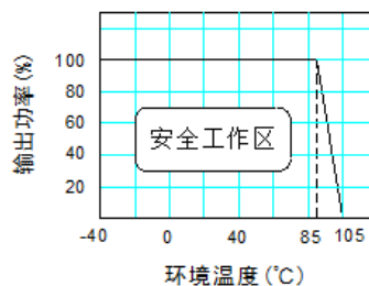
温度曲线图
