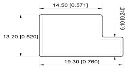
包装管尺寸图
