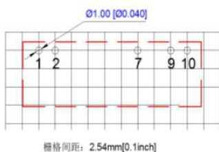
推荐 PCB 图
