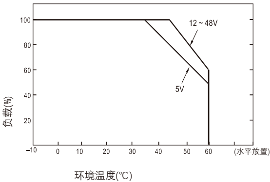
负载减额曲线
