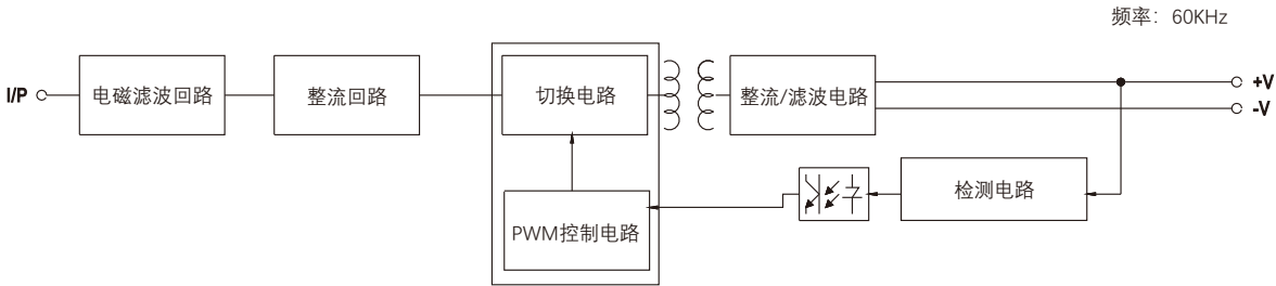
方框图
