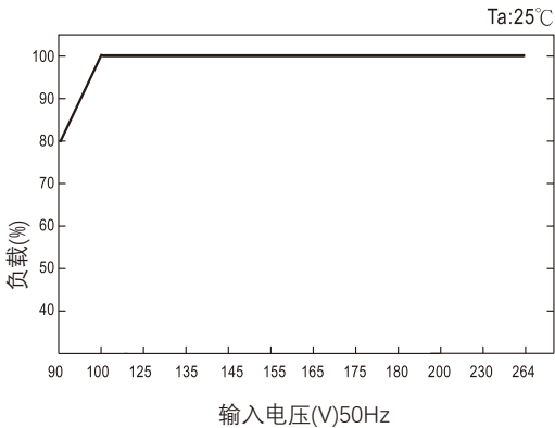
静态特性曲线
