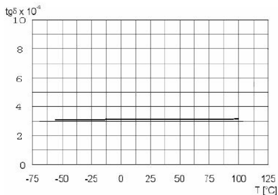
\text{tg}\delta -T
