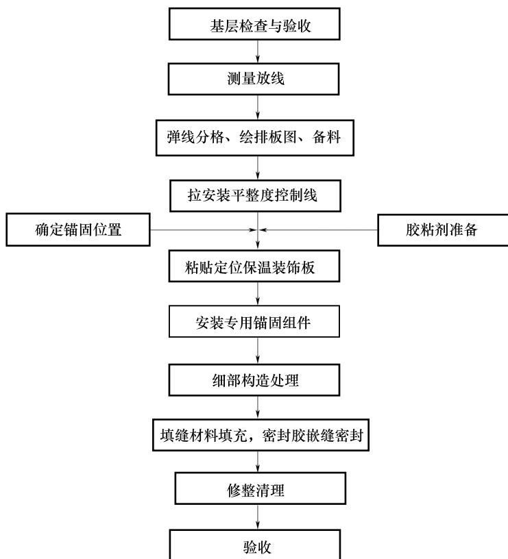
图 6.3.1 施工工序示意图
