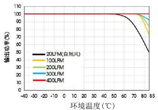
YHWKGS100-48S24S温度降额曲线(Vin=24V)
