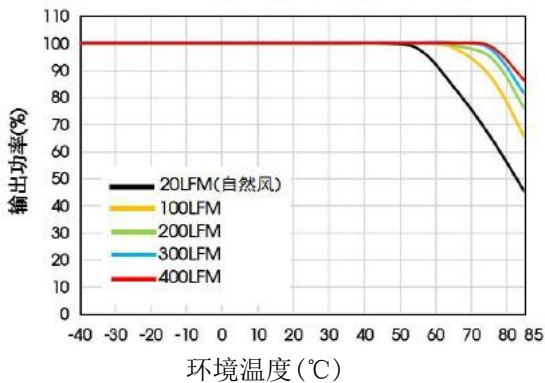
YHWKGS100-48S24温度降额曲线(Vin=24V)
