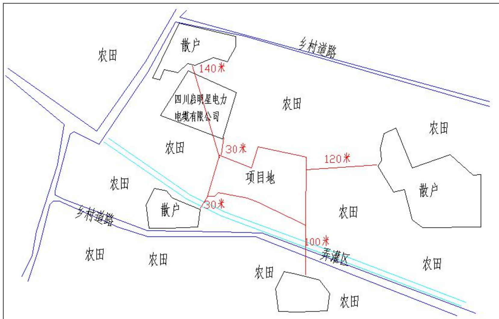
附图 项目外环境关系示意图
