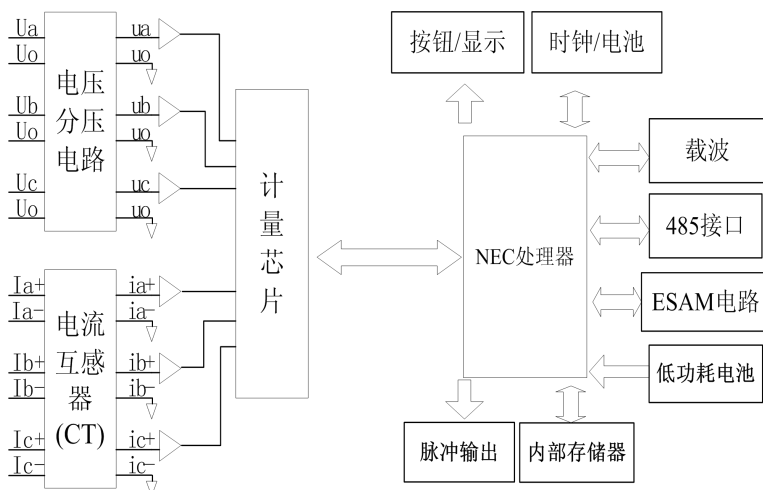
图 1：电能表基本工作原理
