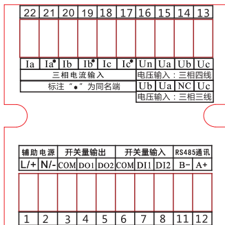
图2：A系列接线图和3系列接线图
