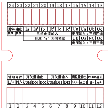
图1：2系列接线图
