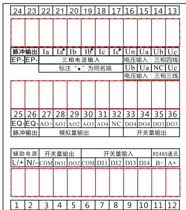
图3：9系列接线图
