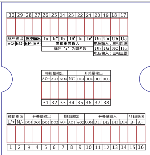
图1：2系列接线图
