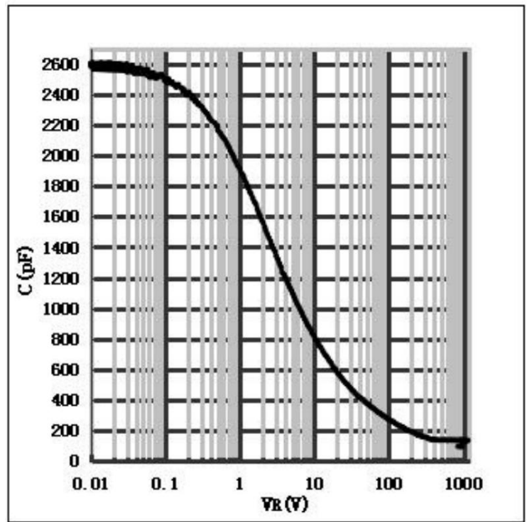
4) 典型电容-反向电压曲线
