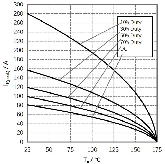
图 4. 电流降额
