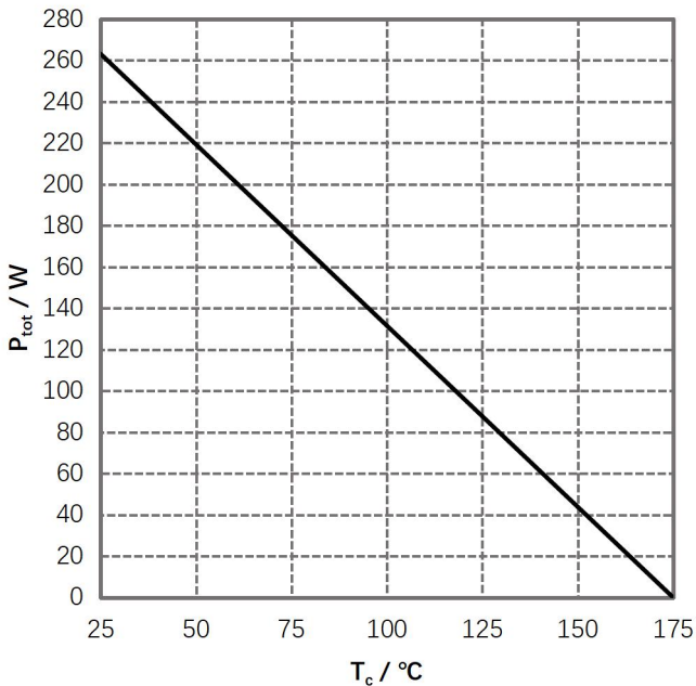
图 3. 功率降低
