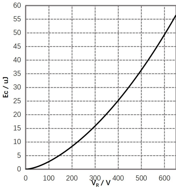
图 7. 电容存储能量
