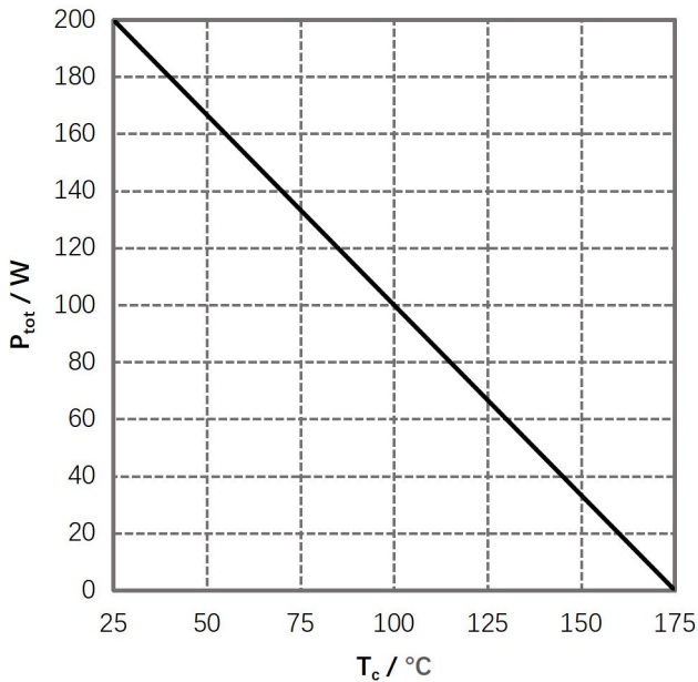
图 3. 功率降低
