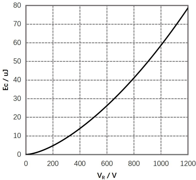
图 7. 电容存储能量
