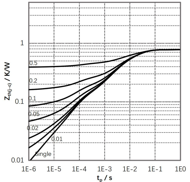
图 8. 瞬态热阻抗
