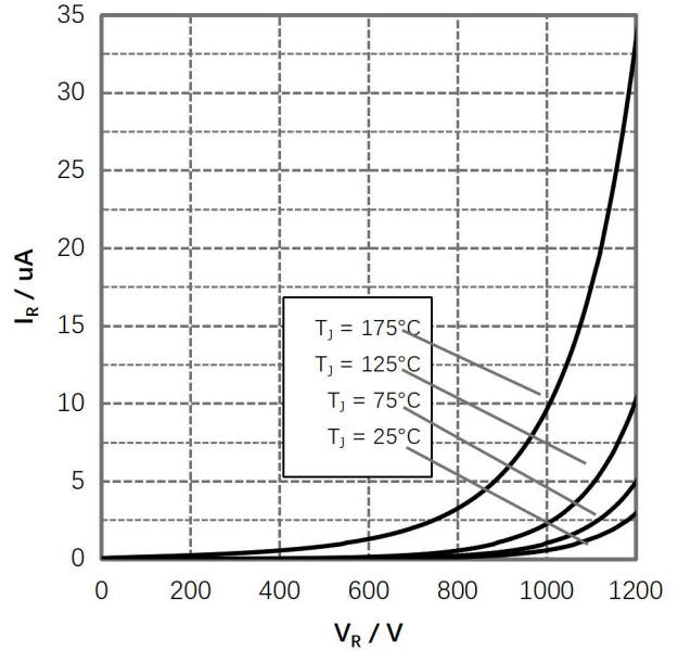
图 2. 反向特性
