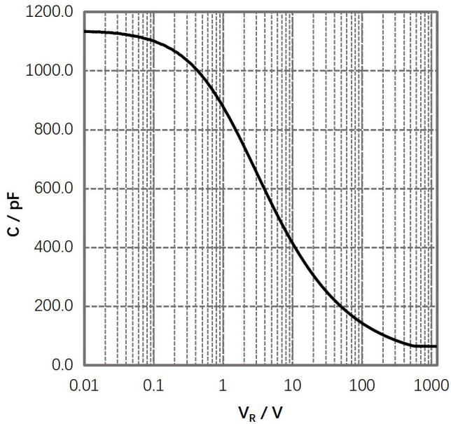
图 5. 电容-反向电压
