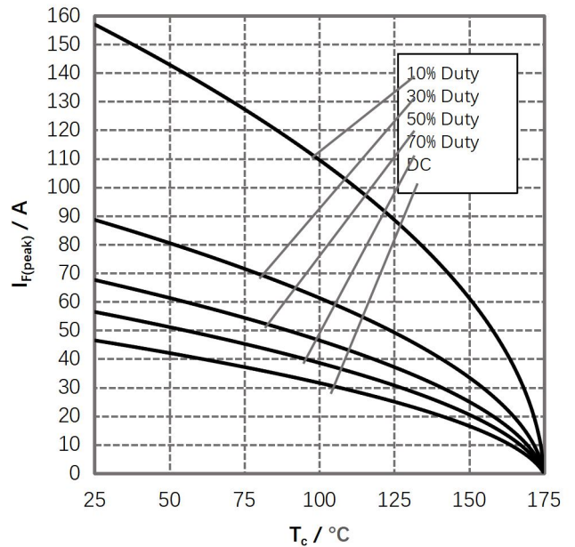
图 4. 电流降额
