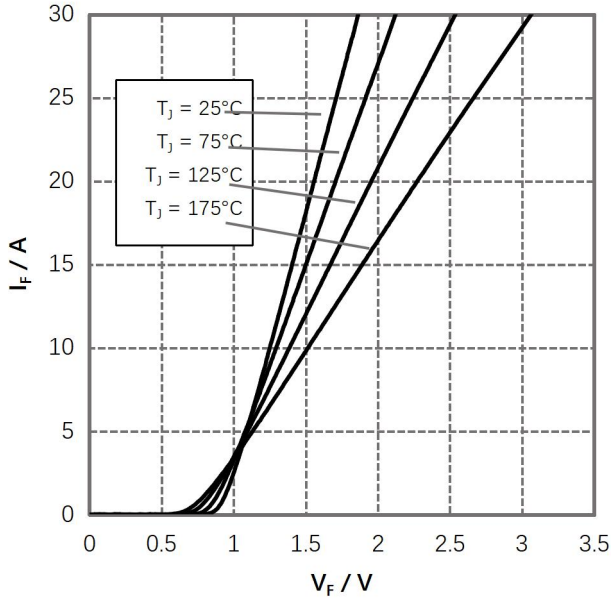
图 1. 正向特性
