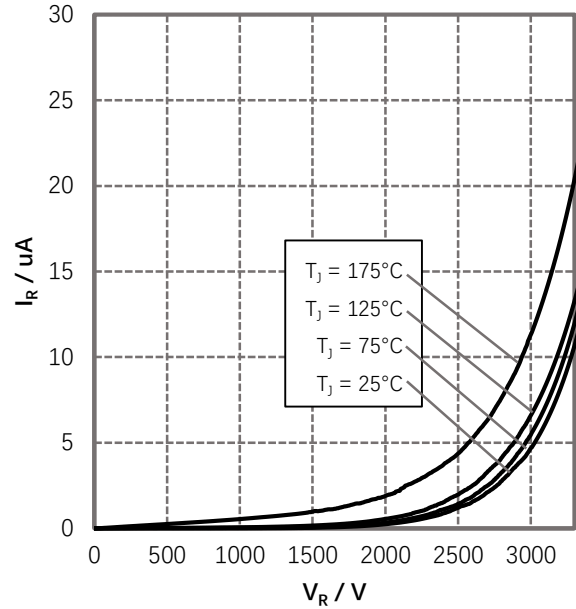
图 2. 反向特性
