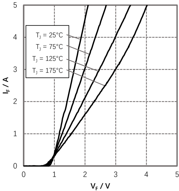
图 1. 正向特性
