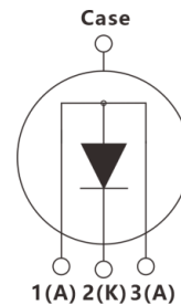
内部电路
