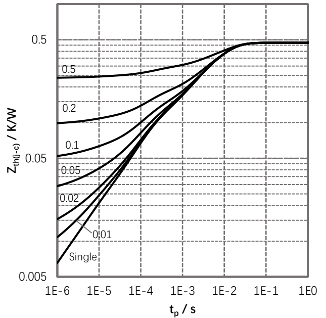
图 8. 瞬态热阻抗
