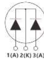
内部电路
