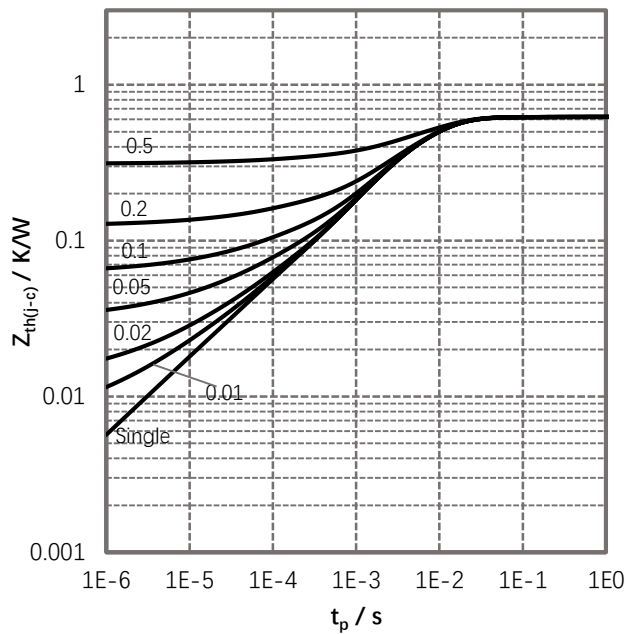
图 8. 瞬态热阻抗
