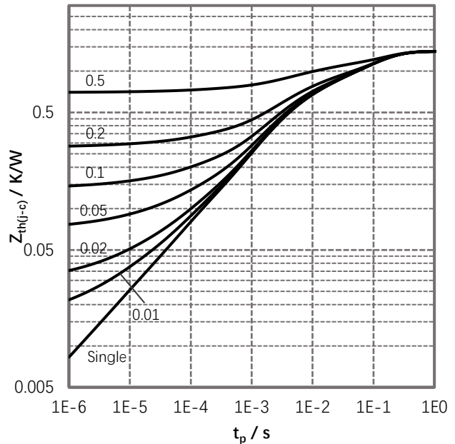
图 8. 瞬态热阻抗
