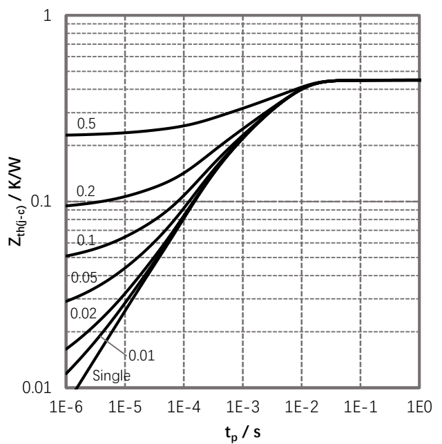
图 8. 瞬态热阻抗
