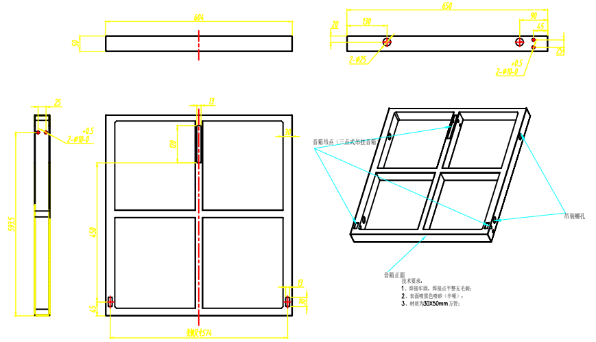
线阵三视图与大架三视图
