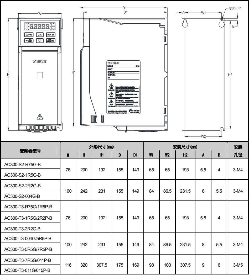
变频器外形尺寸（塑壳）
