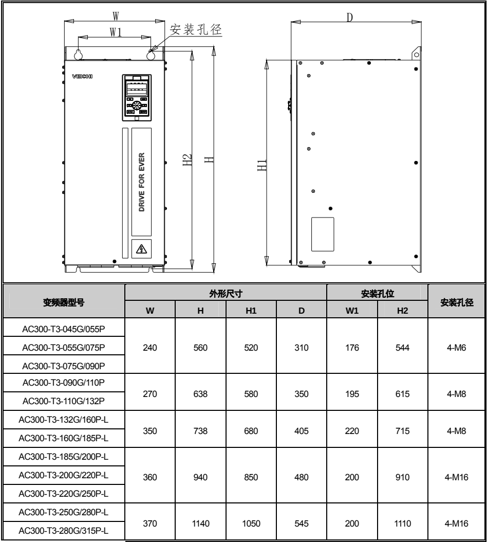
变频器外形尺寸 (铁壳)
