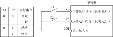
0:两线制控制1示意图
