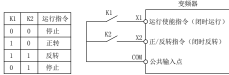
1:两线制控制2示意图
