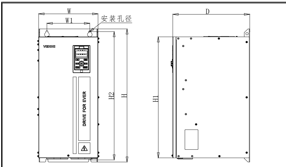
变频器外形尺寸 (铁壳)
