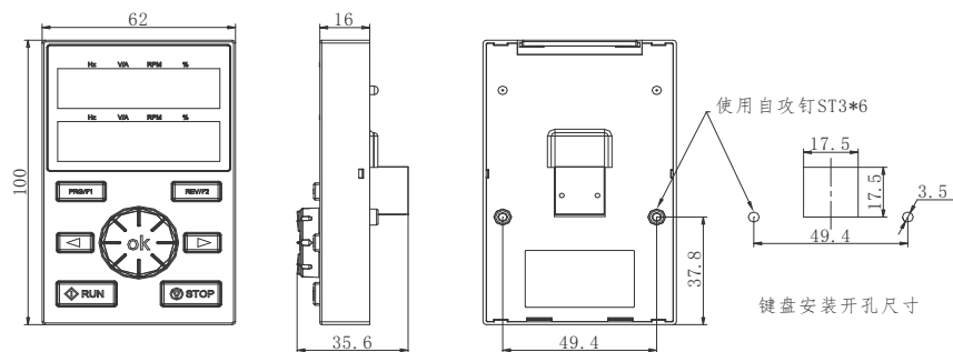
AC310 系列外引键盘外形及开孔尺寸
