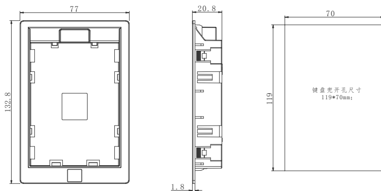
AC310 系列外引键盘外形及开孔尺寸
