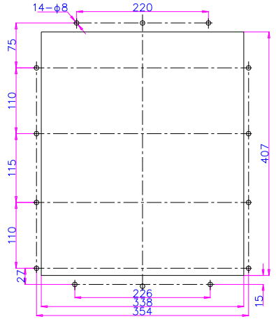
18.5KW-30KW 安装固定开孔图
