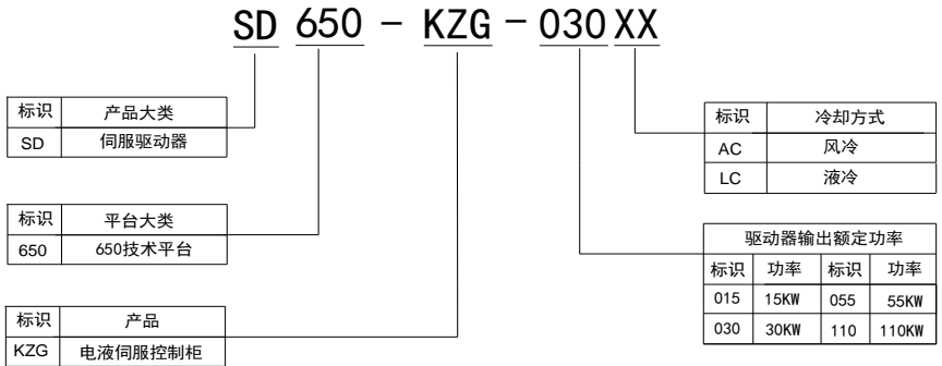
图 2-2：SD650 系列伺服驱动器铭牌含义及命名规则
