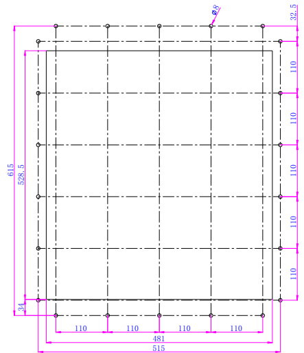
75KW-110KW 安装固定开孔图
