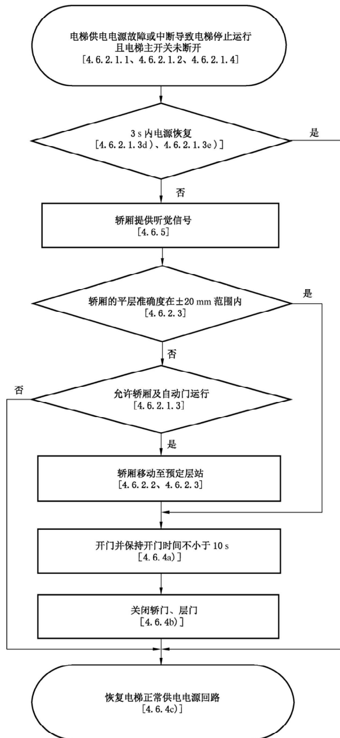
图 A.1 典型的电梯自动救援操作流程
