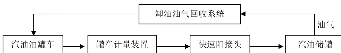
图 2.2-2 汽油卸油工艺流程示意简图
