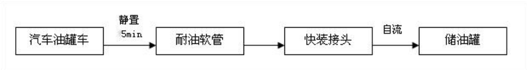
图 2.2-1 柴油卸油工艺流程示意简图
