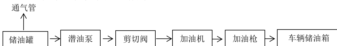
图 2.2-3 柴油加油工艺流程示意简图
